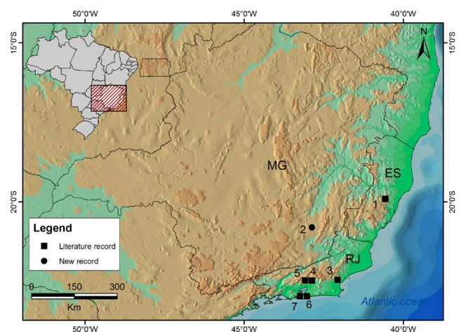
FIGURE 1. Geographic distribution of Trechona venosa Latreille, 1832. ES, state of Espírito Santo; MG, state of Minas Gerais; RJ, state of Rio de Janeiro. Municipalities: 1, Santa Teresa; 2, Viçosa; 3, Casimiro de Abreu; 4, Cachoeiras de Macacu; 5, Petrópolis; 6, Niterói and 7, Rio de Janeiro.
