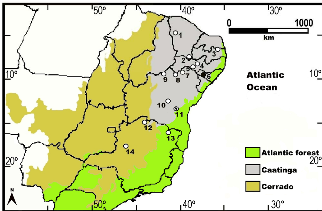
Figure 2. Physalaemus cicada distribution map. New record (black circle) – state of Alagoas (AL): São José da Tapera (6). Literature records (star and white circles) – state of Ceará (CE): Nova Russas (1) (Loebmann and Mai 2008), Brejo Santo (2) (Nascimento et al. 2005); state of Paraíba (PB): Araruna (3) (Arzabe et al. 2005); state of Pernambuco (PE): Betânia (4) (Borges-Nojosa and Santos 2005), Floresta (5) (Borges-Nojosa and Santos 2005); state of Bahia (BA): Curaçá (7) (Nascimento et al. 2005), Juazeiro (8) (Nascimento et al. 2005), Carnaíba (9) (Nascimento et al. 2005), Lençóis (10) (Santana and Juncá 2007), Maracás, type locality (11) (Bokermann 1966); state of Minas Gerais (MG): Matias Cardoso (12) (Nascimento et al. 2005), Pedra Azul (13) (Nascimento et al. 2005), João Pinheiro (14) (Silveira 2006).
